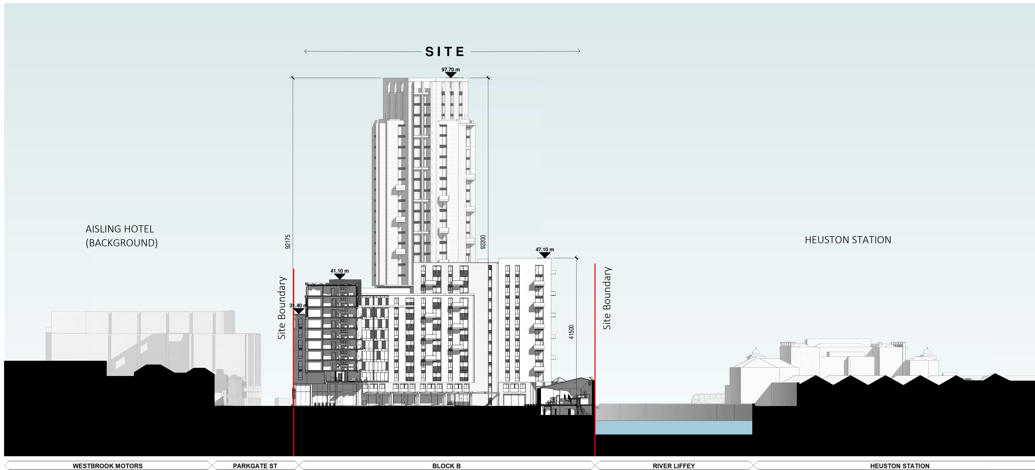
Contiguous Section 2 - 2 1 : 500
